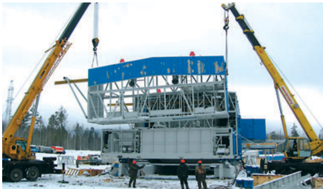
Демонтаж буровой установки на скважине № 2 Абаканской для Дулисьминского НГКМ.
